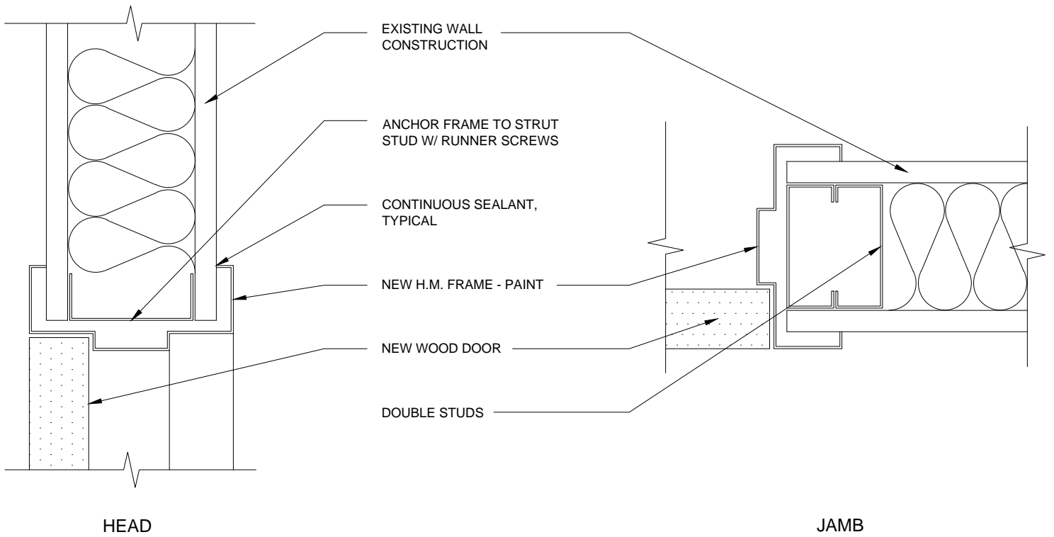
1 HEAD/JAMB DETAILS SCALE: 3" = 1'-0"
